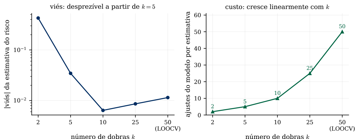
Figura 3: Estimativa do risco de um polinômio de grau 5 sobre n = 50 pontos, repetida em 300 amostras independentes. À esquerda, o viés da estimativa (escala logarítmica): com k = 2 ele é desastroso — treinar com 25 pontos é coisa muito diferente de treinar com 50 — e a partir de k = 5 já é desprezível. À direita, o custo, que cresce linearmente: a LOOCV pede dez vezes mais ajustes que k = 5 .
